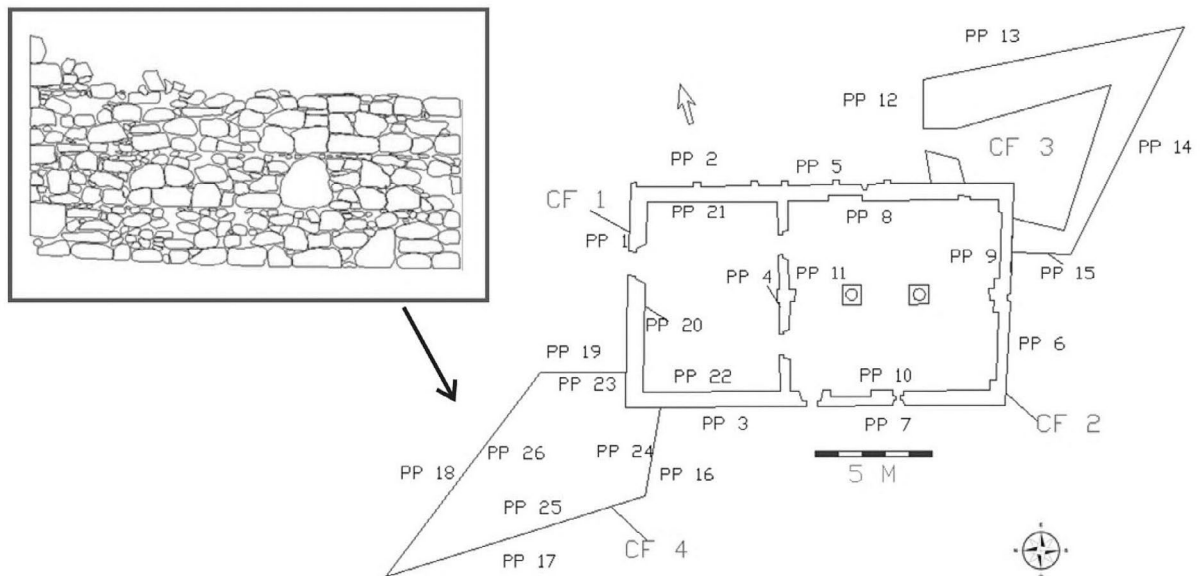
Figura 9. tipo murario IV di San Piero in Campo e localizzazione in pianta.
