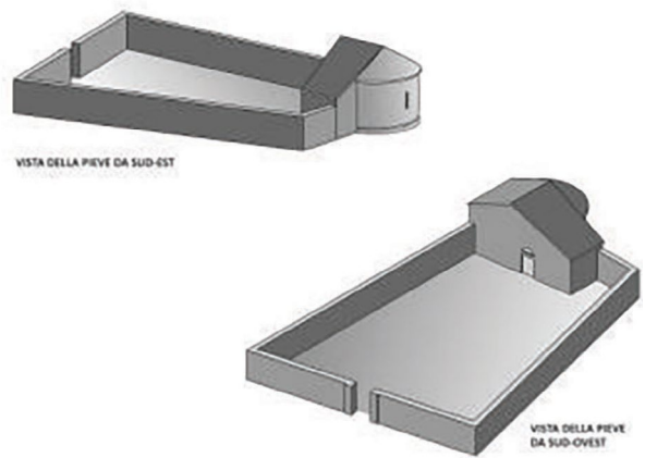
Figura 62. Rilievo geometrico di San Michele di Capoliveri realizzato da I.Trifirò, I.Costantino, M.Grassini.
