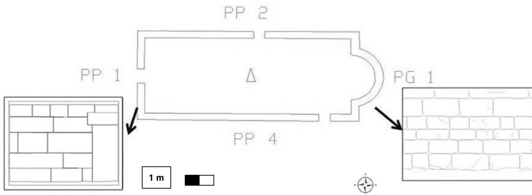
Figura 10. Pianta di San Giovanni con l'indicazione dei prospetti.
