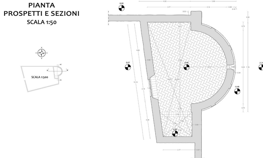
Figura 19. Pianta di San Michele.
