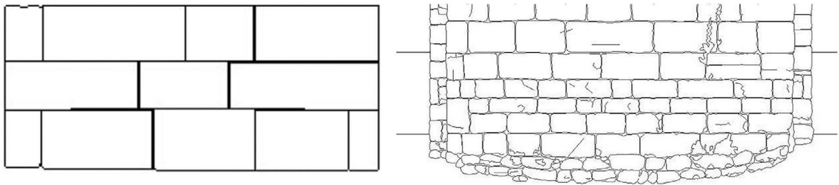
Figura 4. tipo murario 1 (sinistra) e tipo murario 2 (destra).
