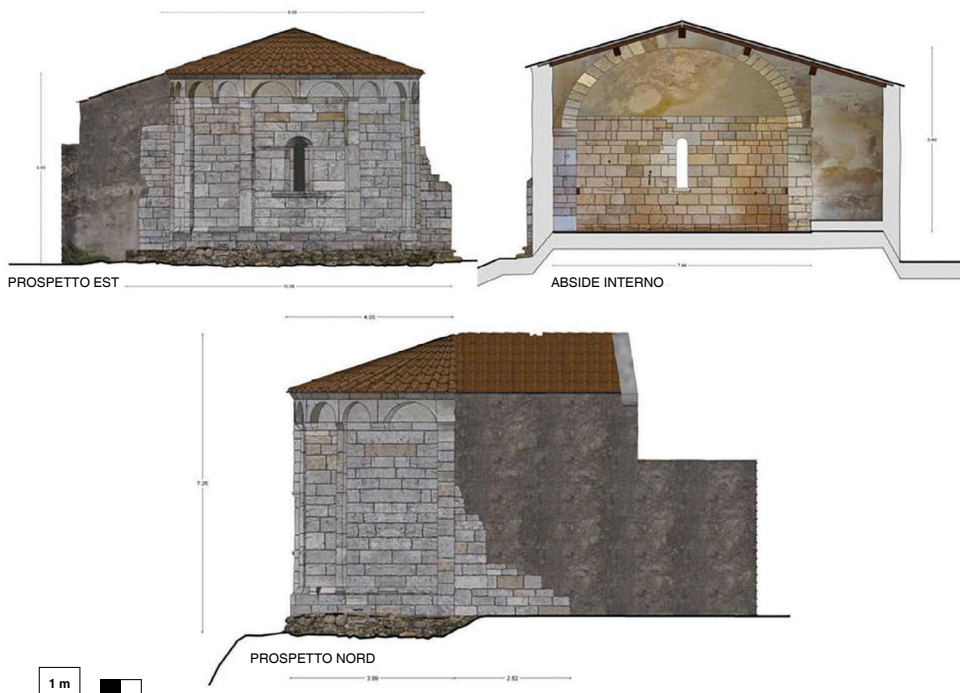
Figura 20. Rilievi di San Michele a Capoliveri realizzati da I. Costantino, I. Trifirò e M. Grassini.
