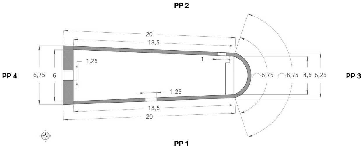
Figura 3. Pianta di San Lorenzo con l'indicazione dei prospetti (PP) e localizzazione dei tipi murari.
